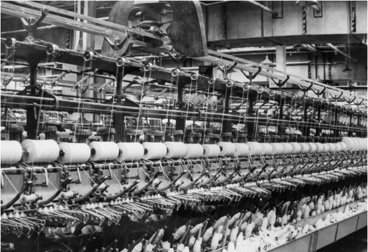
Одна из тростильных машин Дедовской кордной фабрики. Конец 1950-х годов
