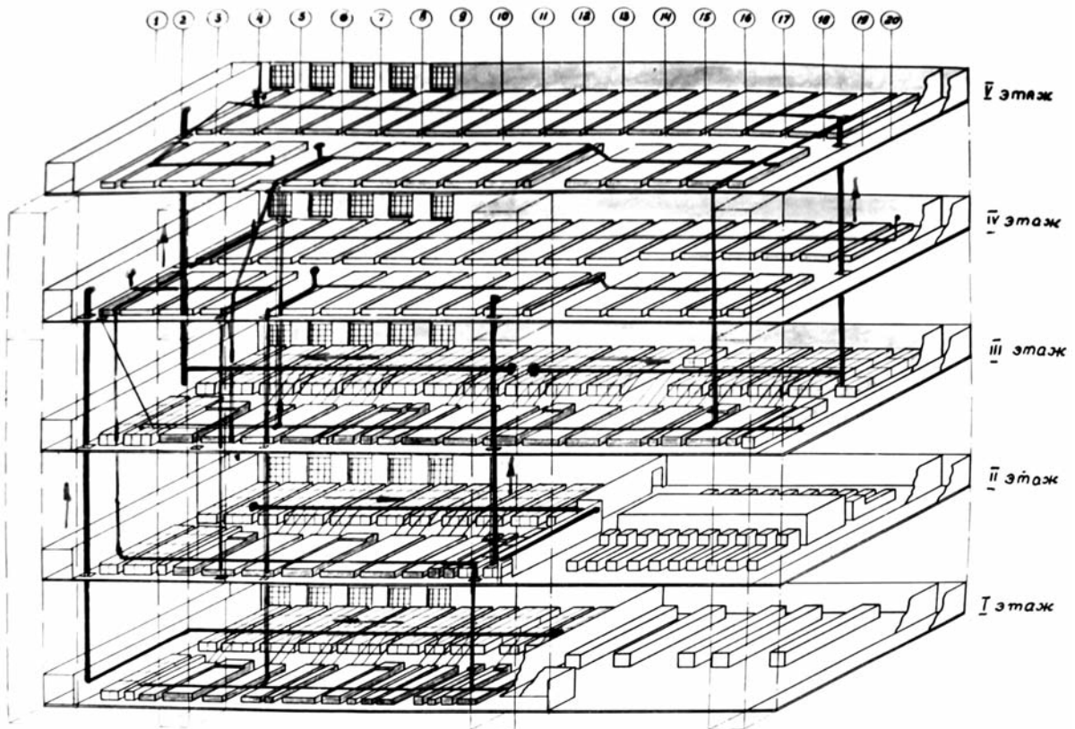
Схема бестарной транспортировки материалов на Дедовской кордной фабрике. Конец 1950-х годов
